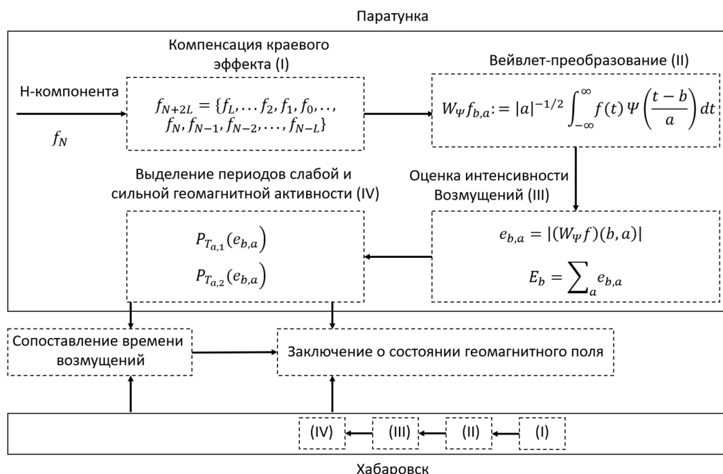
Рис. 3. Схема оценки состояния геомагнитных данных. [Figure 3. Geomagnetic data state estimation scheme.]
