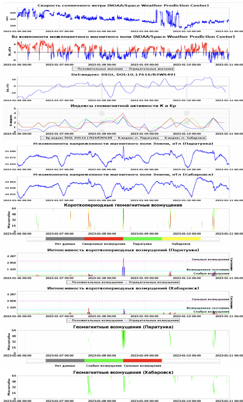
Рис. 5. Результаты работы геомагнитной компоненты системы «Аврора» в период 06–10 января 2023 г.
