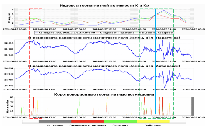
Рис. 7. Результаты работы системы «Аврора» в период 26-28 июня 2024 г. [Figure 7. «Aurora» system results for the period 26-28 June 2024.]
