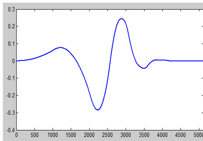
Рис. 1. Вейвлет Добеши порядка 3. [Figure 1. Dobeshi wavelet of order 3.]
