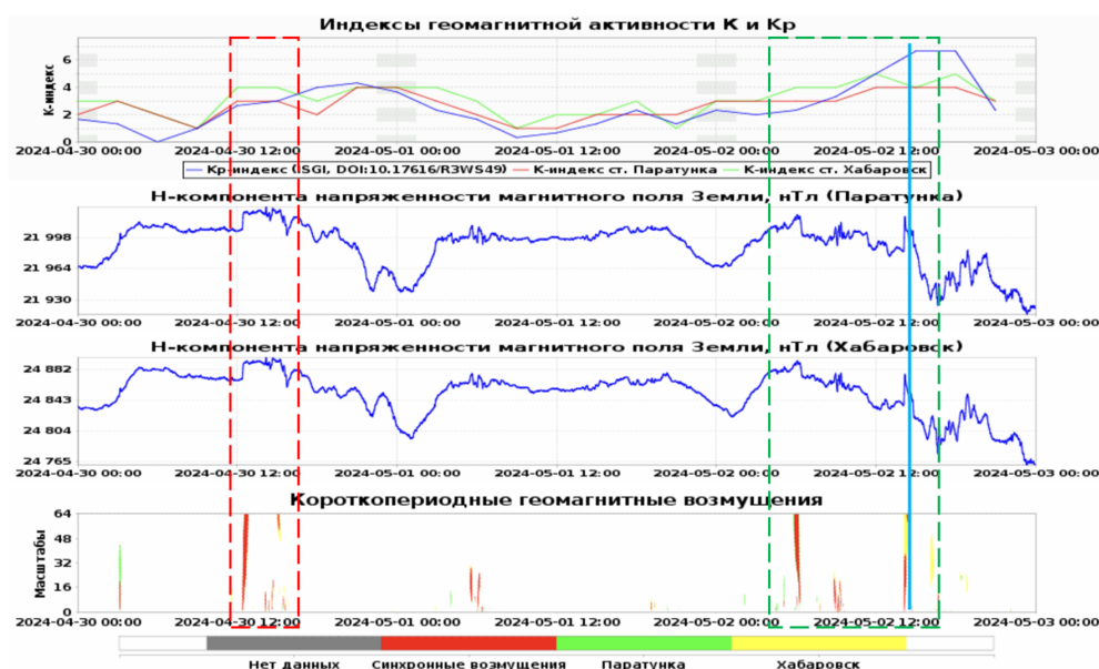
Рис. 6. Результаты работы системы «Аврора» в период 30 апреля – 02 мая 2024 г. [Figure 6. «Aurora» system results for the period 30 April – 02 May 2024.]
