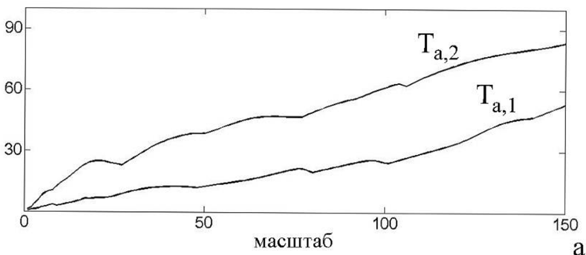
Рис. 2. Результаты расчета пороговых значений T_{a,1} и T_{a,2} . На оси ox отмечены масштабы a , на оси oy - значения T_{a,1} и T_{a,2} .
