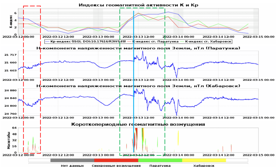
Рис. 8. Результаты работы системы «Аврора» в период 12-14 марта 2022 г.
