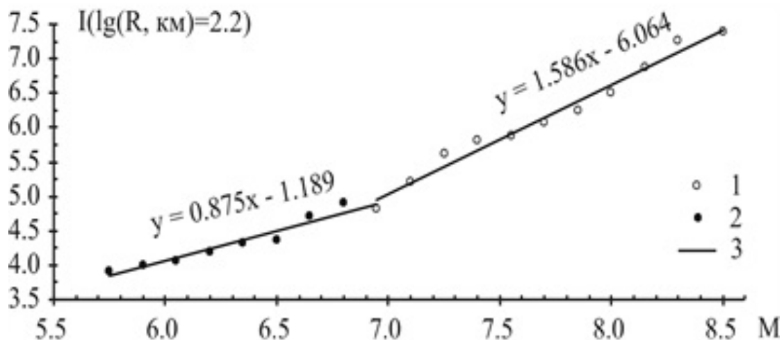
Рис. 4. График значений интенсивности сейсмического воздействия I в средней точке интерполяционных изолиний (рис. 3) при различных значениях магнитуд M : 1 – значения сейсмической интенсивности I для средних точек ( \lg(R) = 2.2 ) интерполяционных изолиний (рис. 3) при различных значениях магнитуды M землетрясений с M \geq 7.0 ; 2 – то же для землетрясений с M < 7.0 ; 3 – линии аппроксимации зависимостей для каждого из двух указанных диапазонов
