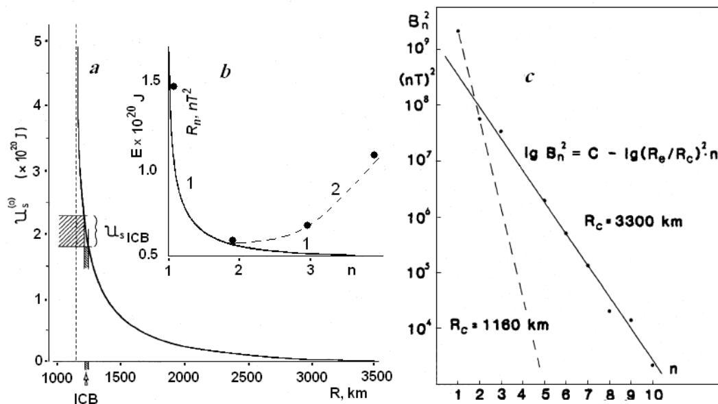
Рис. 4. Оценка величины энергии геомагнитного поля в зависимости от радиуса Земли (а) [9], от номера сферической гармоники (b) для поверхности внутреннего ядра, спектр геомагнитного поля (c) для двух поверхностей радиусом R_c [10]
